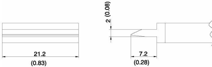
T7-1403 Spatula 21.2
