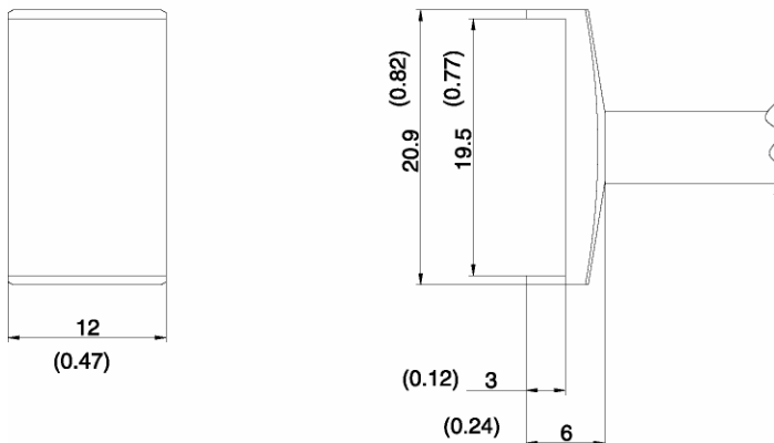
T7-1010 SOP 19.5×12
