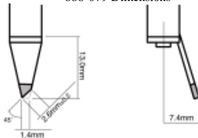
888-079 Dimensions
