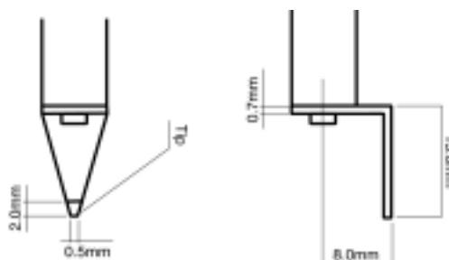
888-080 Dimensions
